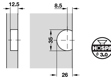
boormaten in de bodem en in de klep
