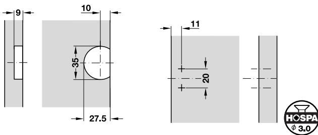
boormaten in de klep
