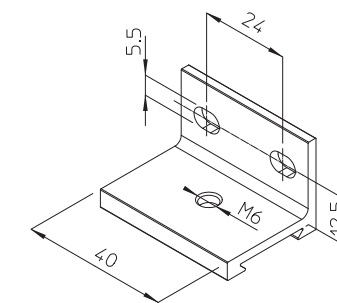
Staffa per binario tipo 2-3 Interasse staffe di ancoraggio min. 300 - max 400
